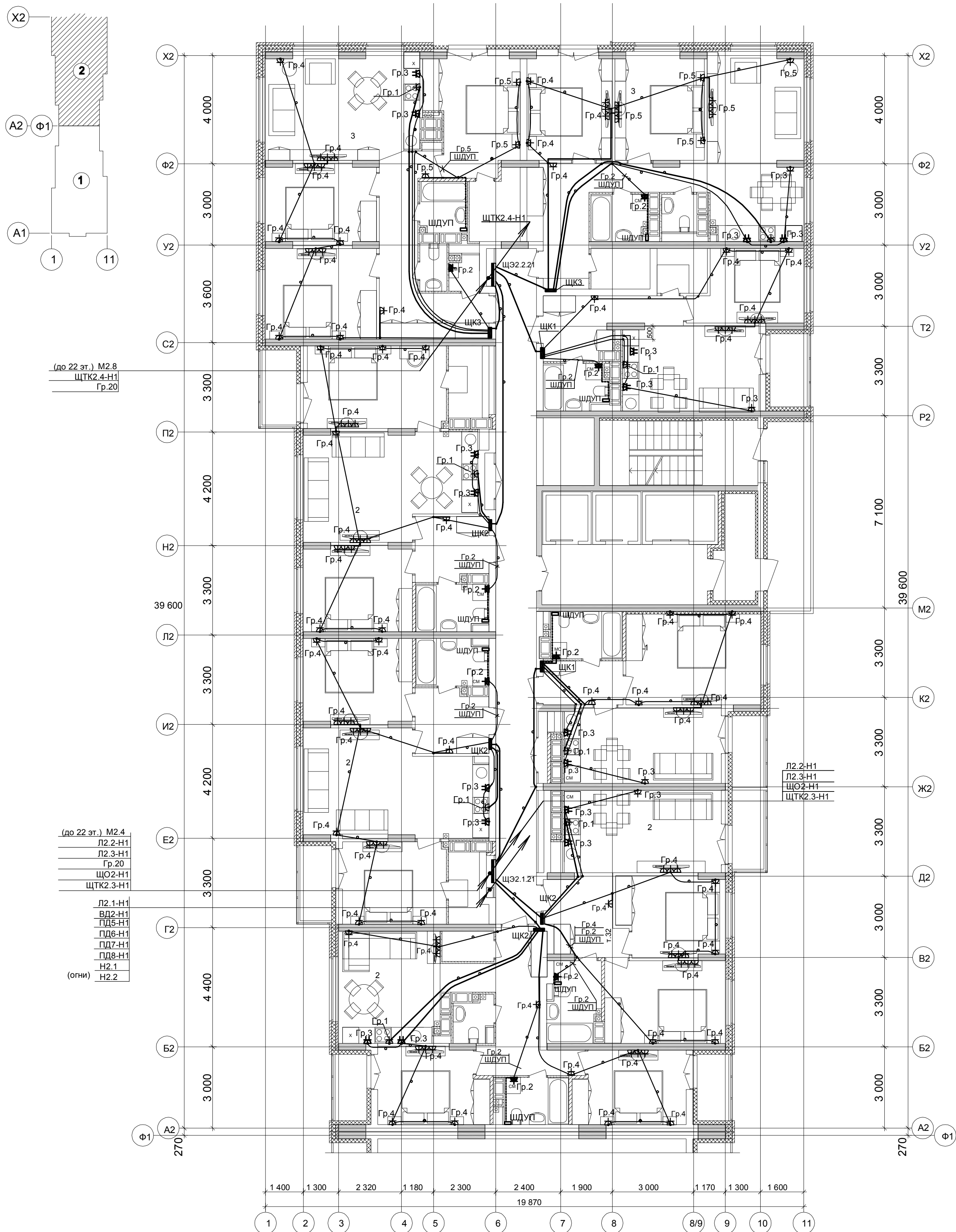
План 22 этажа.
